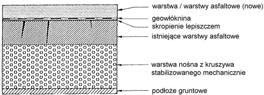
Rys. 3. Wzmocnienie nawierzchni asfaltowej z warstwą profilującą
